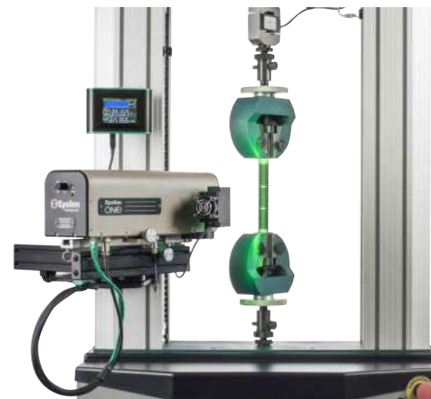
非接觸式延伸計
