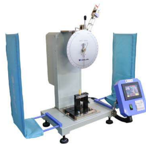
Charpy/Izod試驗機
